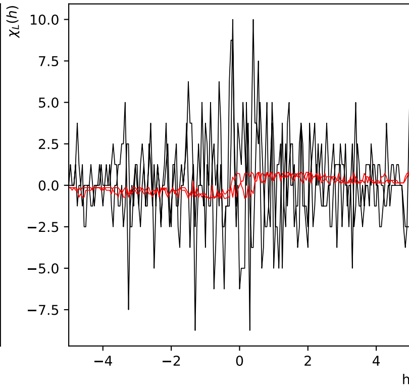
\chi_L(h) réseau de taille L=4 à T=5
