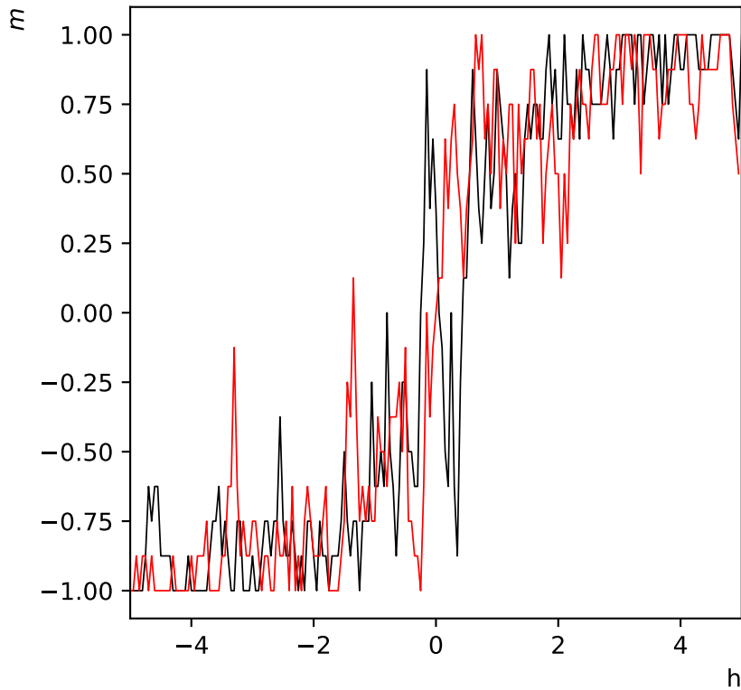
Hystérésis de l'aimantation réseau de taille L=4 - h=5 à T=5
